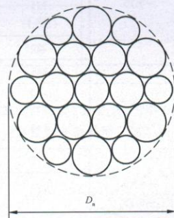
图 5 1×19 结构瓦林忒式钢绞线外形示意图
