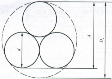
图 2 1×3 结构钢绞线外形示意图
