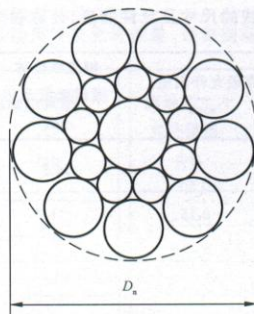
图 4 1×19 结构西鲁式钢绞线外形示意图
