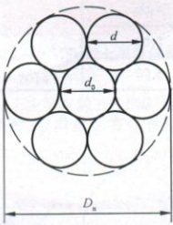
图 3 1×7 结构钢绞线外形示意图
